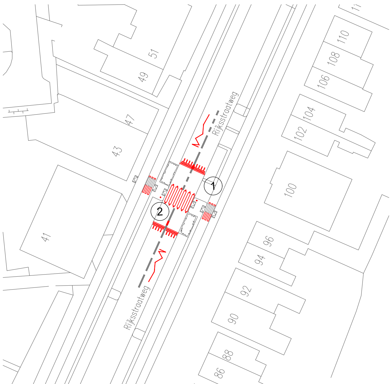
Maatregelen bij voetgangersoversteekplaats ter hoogte van Rijksweg 43 schaal 1:500
