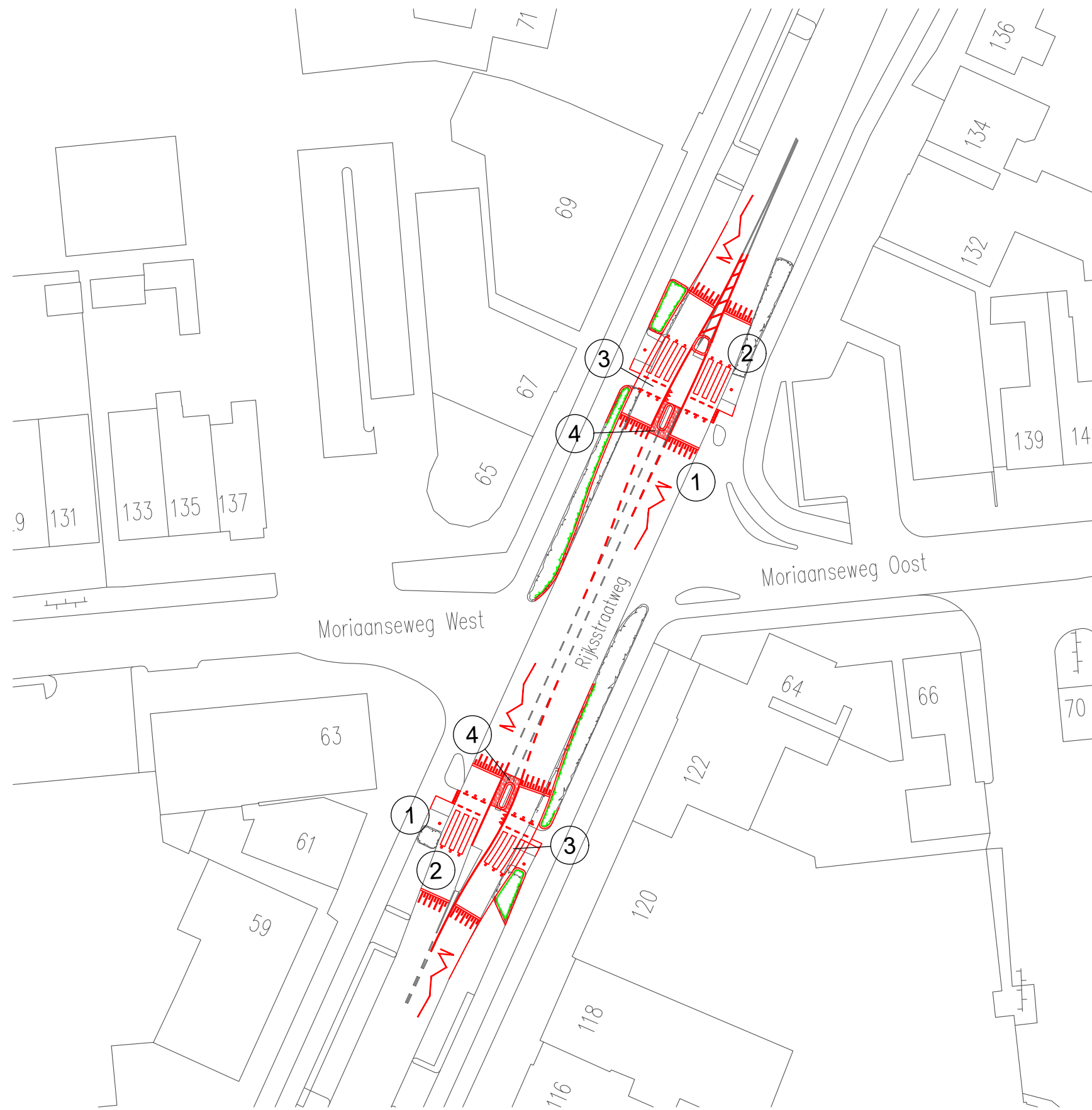
Maatregelen ter plaatse van kruispunt Rijksweg/Moriaanseweg schaal 1:500
