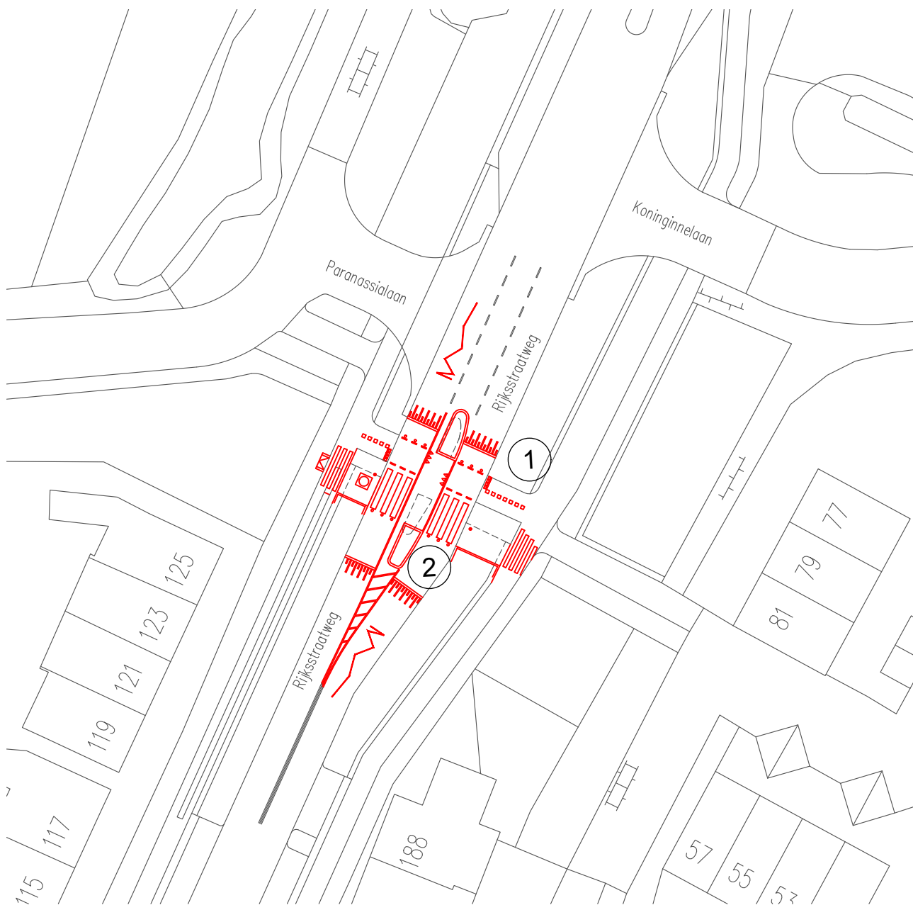
Maatregelen bij voetgangers-/fietsoversteekplaats ter hoogte van Parnassialaan schaal 1:500
