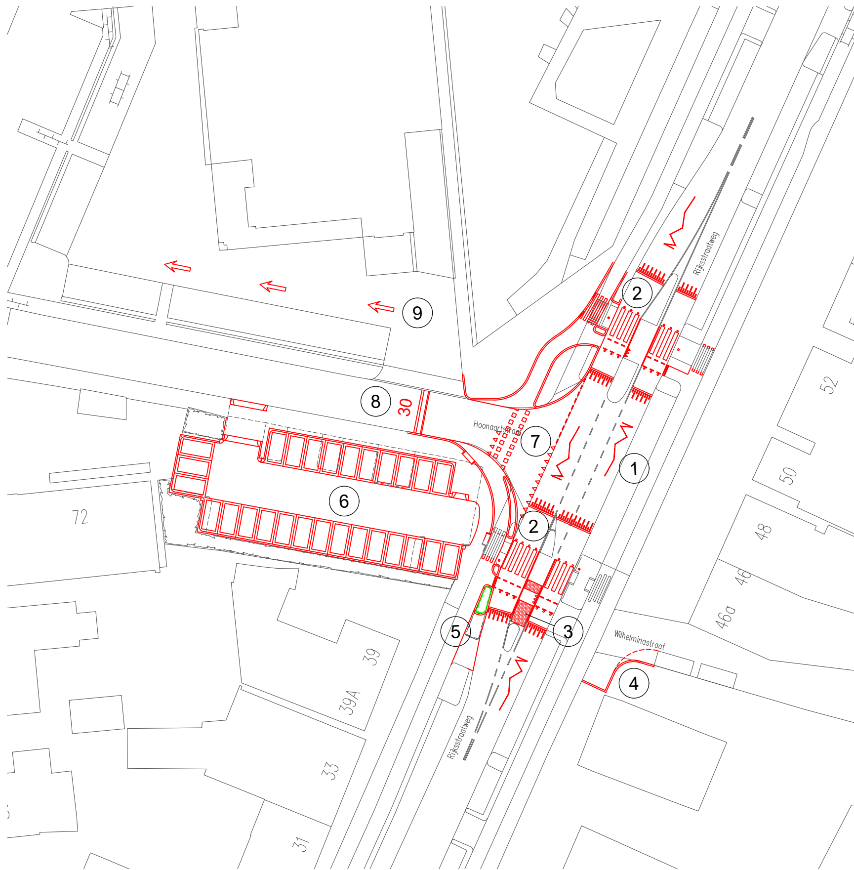
Maatregelen ter plaatse en ter hoogte van kruispunt Rijksstraatweg/Hoonartstraat schaal 1:500
