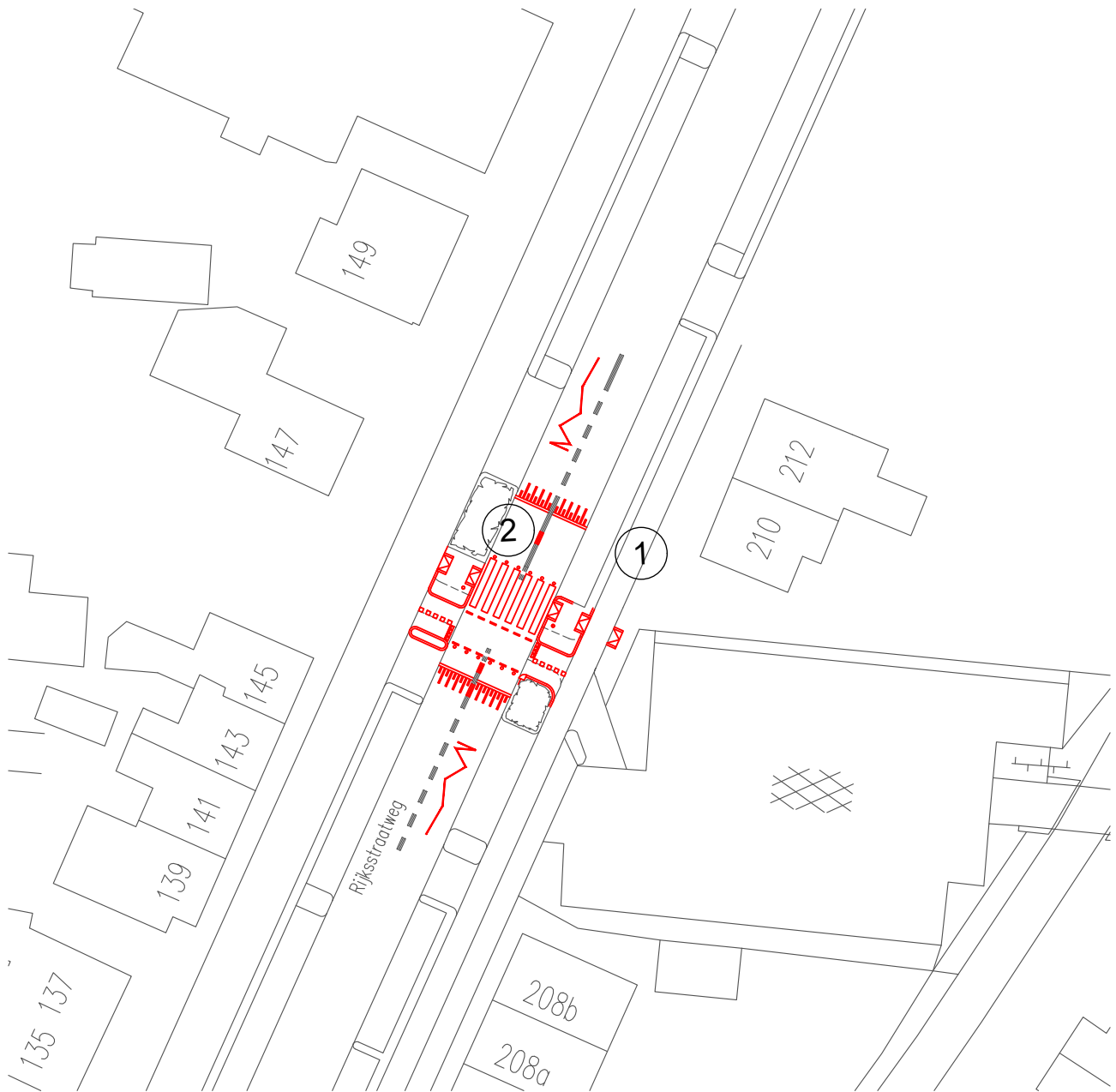
Maatregelen bij voetgangers-/fietsoversteekplaats ter hoogte van Rijsstraatweg 147 schaal 1:500
