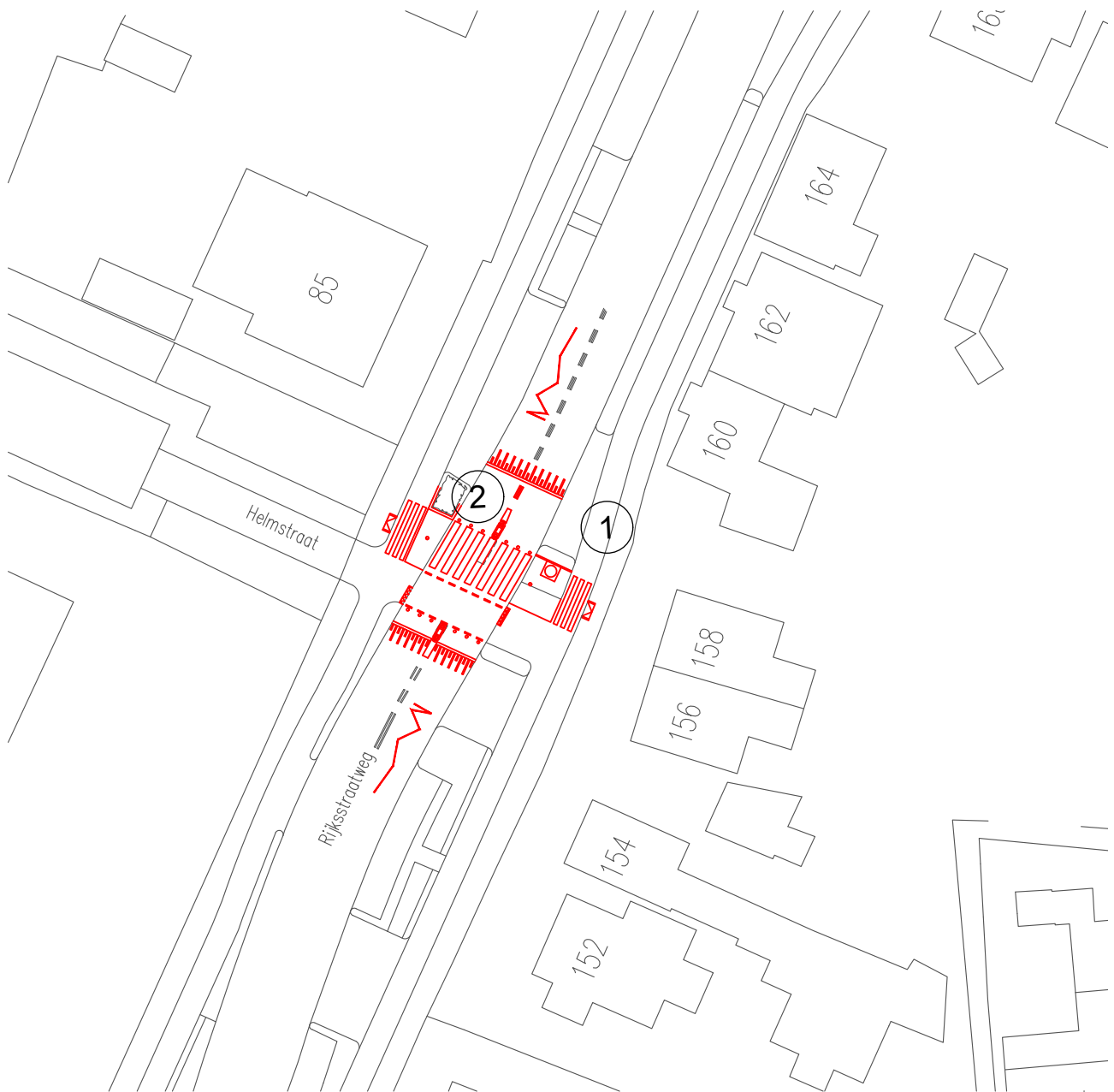
Maatregelen bij voetgangers-/fietsoversteekplaats ter hoogte van Helmstraat schaal 1:500
